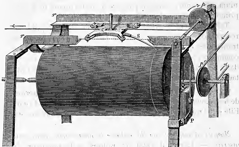
Fig. 124. — Appareil pour inscrire un mouvement rectiligne quelconque.
